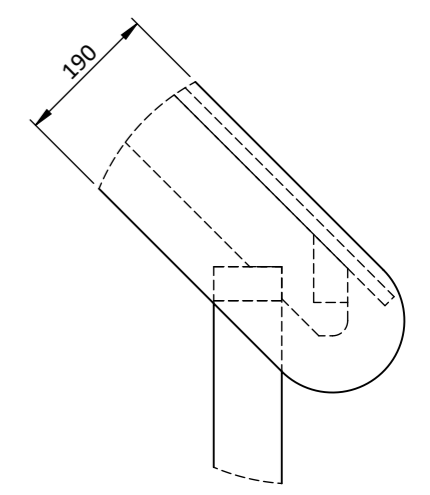
A: 190x45 Barge Board Heel
